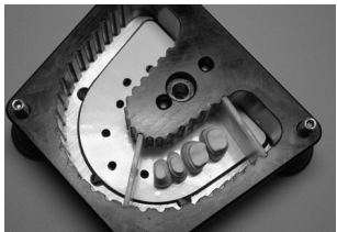
Der Superdub - 3 D Dublierung Bestell-Nr. 10150 -10151
